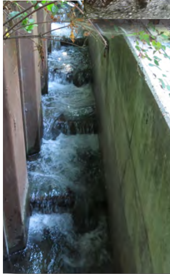
Abbildung 13: Beckenpass des Kraftwerks Sursee (50003) mit einer zu hohen Wasser-spiegeldifferenz beim Ausstieg oben (rechts).
